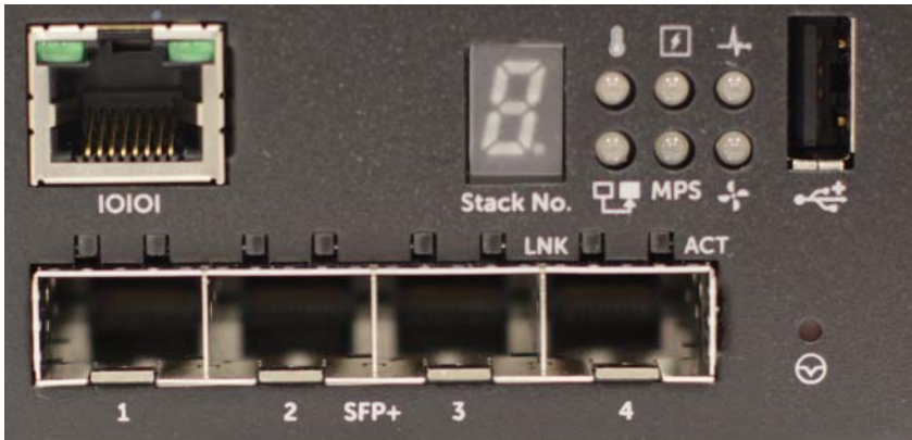
Abbildung 1-3. Dell-Netzwerke N1524P Nahansicht
